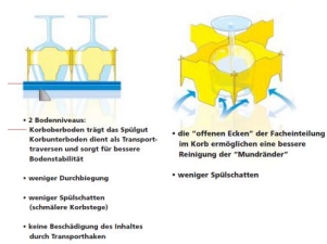
Duplexboden Offene Facheinteilungen
