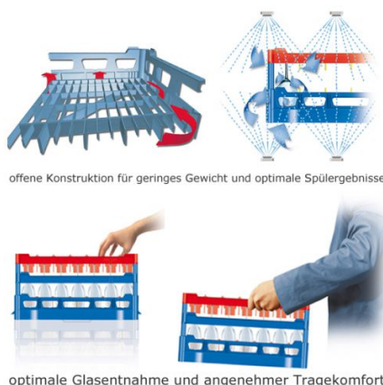
Duplexboden
